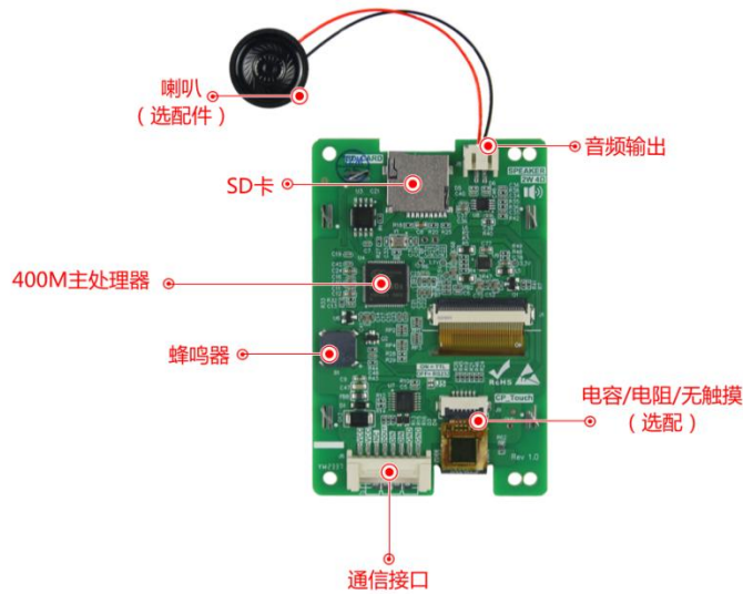
图 1-2 硬件配置图
