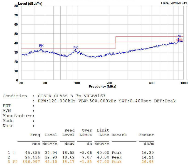
图 5-7 辐射测试垂直方向
